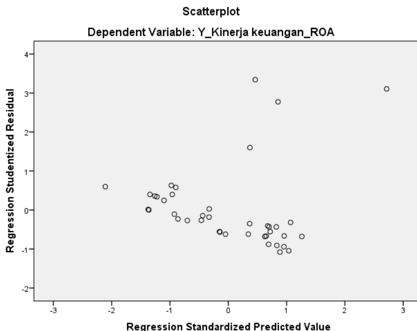
Gambar 1. Diagram Heteroskedastisitas
